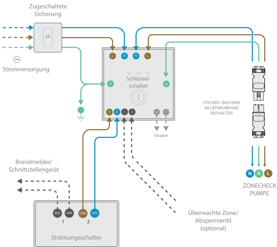
Bild 6: Anschlußplan Zonecheck mit Schlüsselschalter
